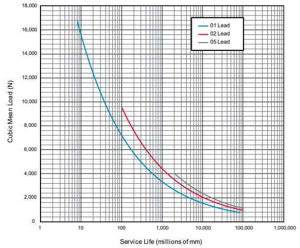
Exlar GTX080
