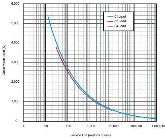
Exlar GTX060
