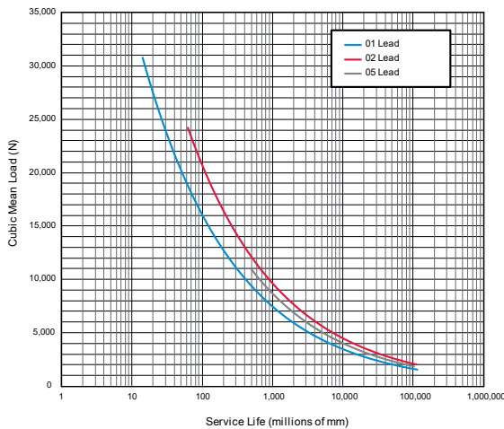
GTX100
